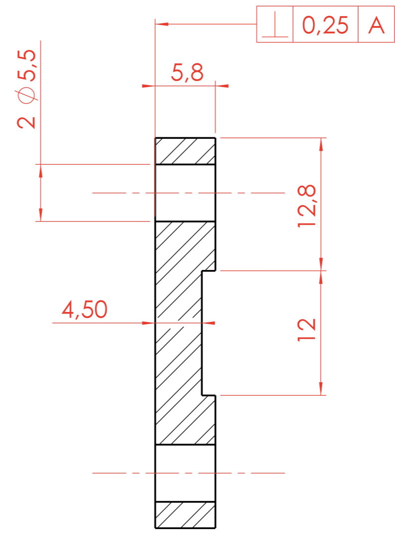
COUPE A-A
